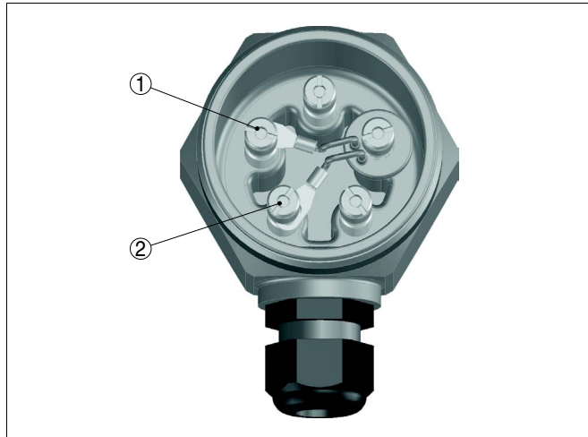
Abb. 6: Montage des Bauteils zur Leitungsbruchüberwachung
