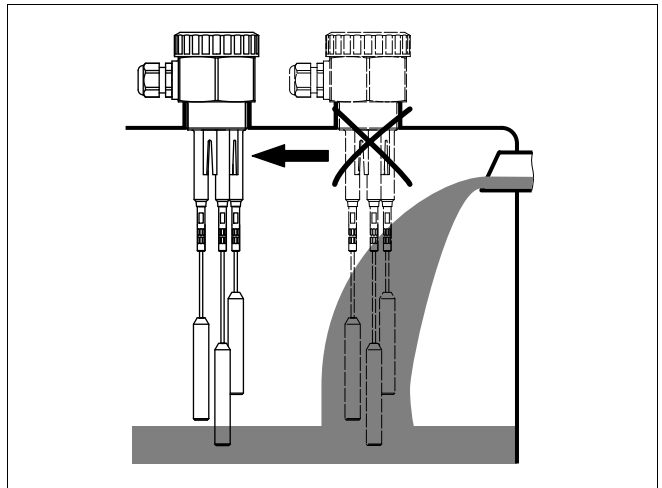
Abb. 3: Einströmendes Füllgut
