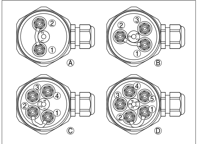
Abb. 4: Anschlussraum der Messsonde - 220 k \Omega -Widerstand zwischen den Klemmen 1 und 2
