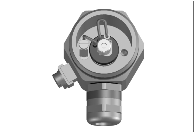
Fig. 7: Montaje del componente para el monitoreo de rotura de línea
