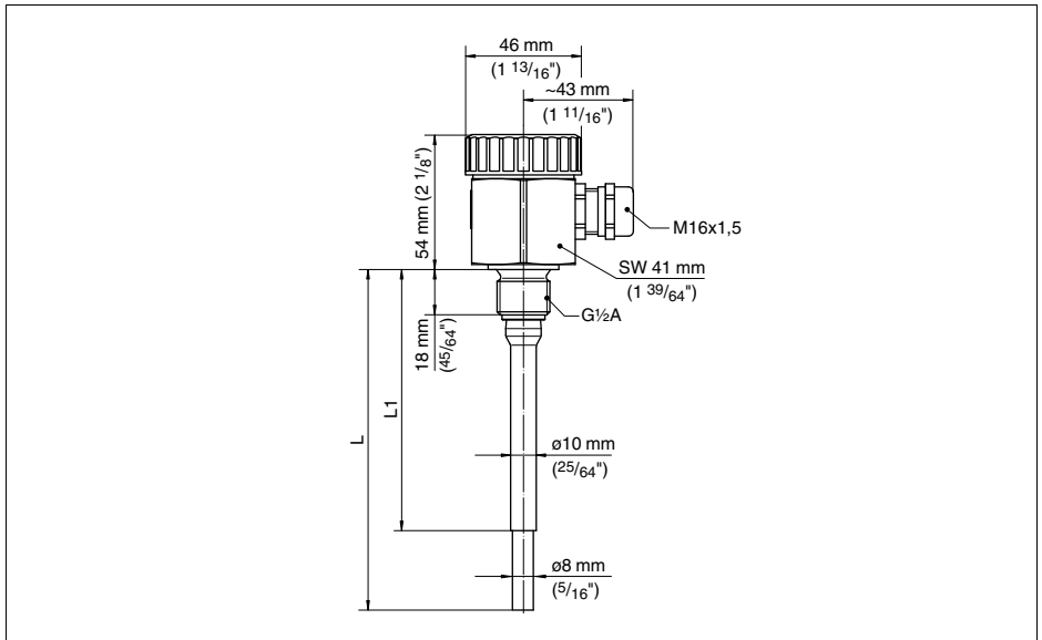
Fig. 8: Sonda de medición de varilla conductiva EL 1
