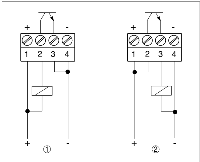
Fig. 6: Electrónica con salida de transistores
