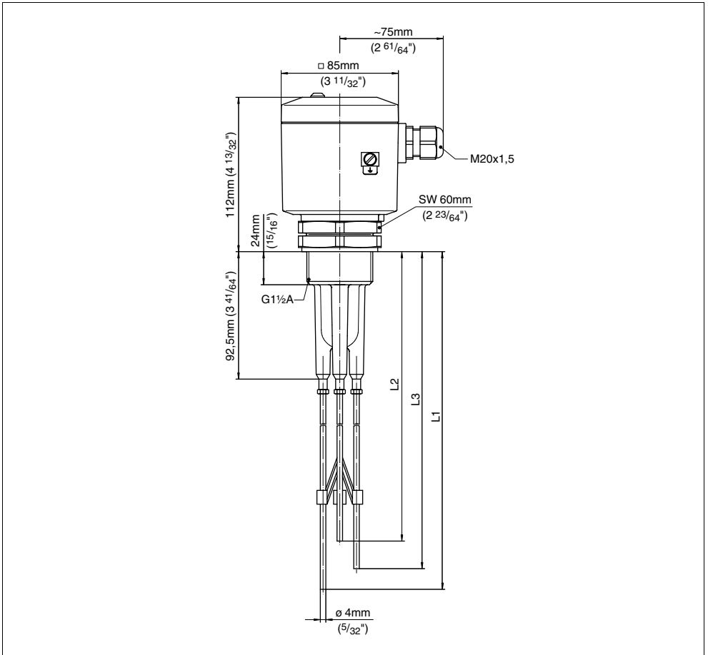
Fig. 17: VEGAKON 66 con tres electrodos
