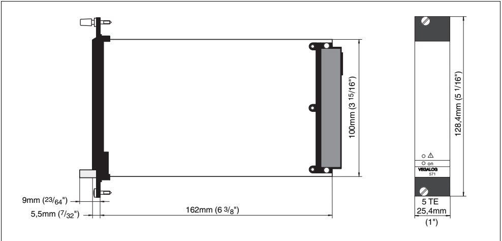
Fig. 5: Encombrement VEGALOG 571 AA
