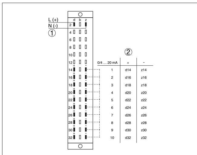
Fig. 3: VEGALOG 571 AA 1)
